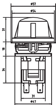
MG1465 E14 (Max.30W; Pin: 90° & 180° available)
